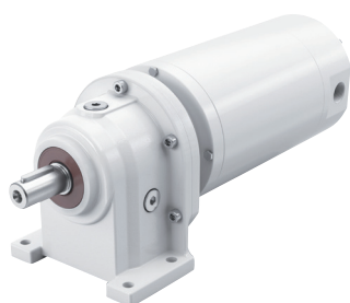
Stirnradgetriebe mit Glattmotor Aluminum SBA
